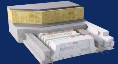
Plancher Terrawatt avec Isorupteurs dB
