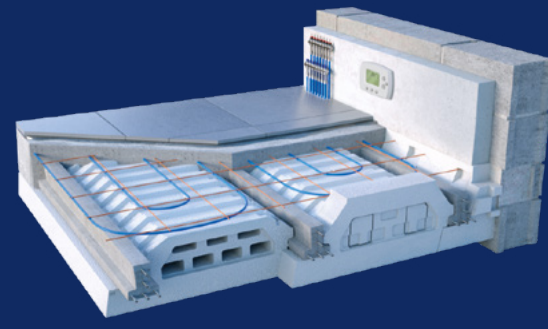
Plancher Milliwatt et Plancher Milliwatt Chauffant / Rafrâichissant
