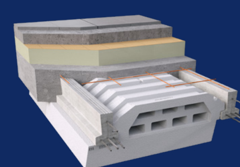
Plancher Duo Isoleader et chape flottante
