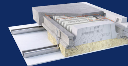
Plancher Silence avec Isorupteurs dB ou Isorupteurs dB EI30
