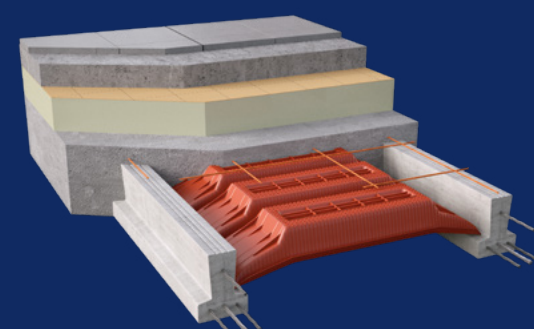
Plancher EcoVS ou Plancher EMR et chape flottante
